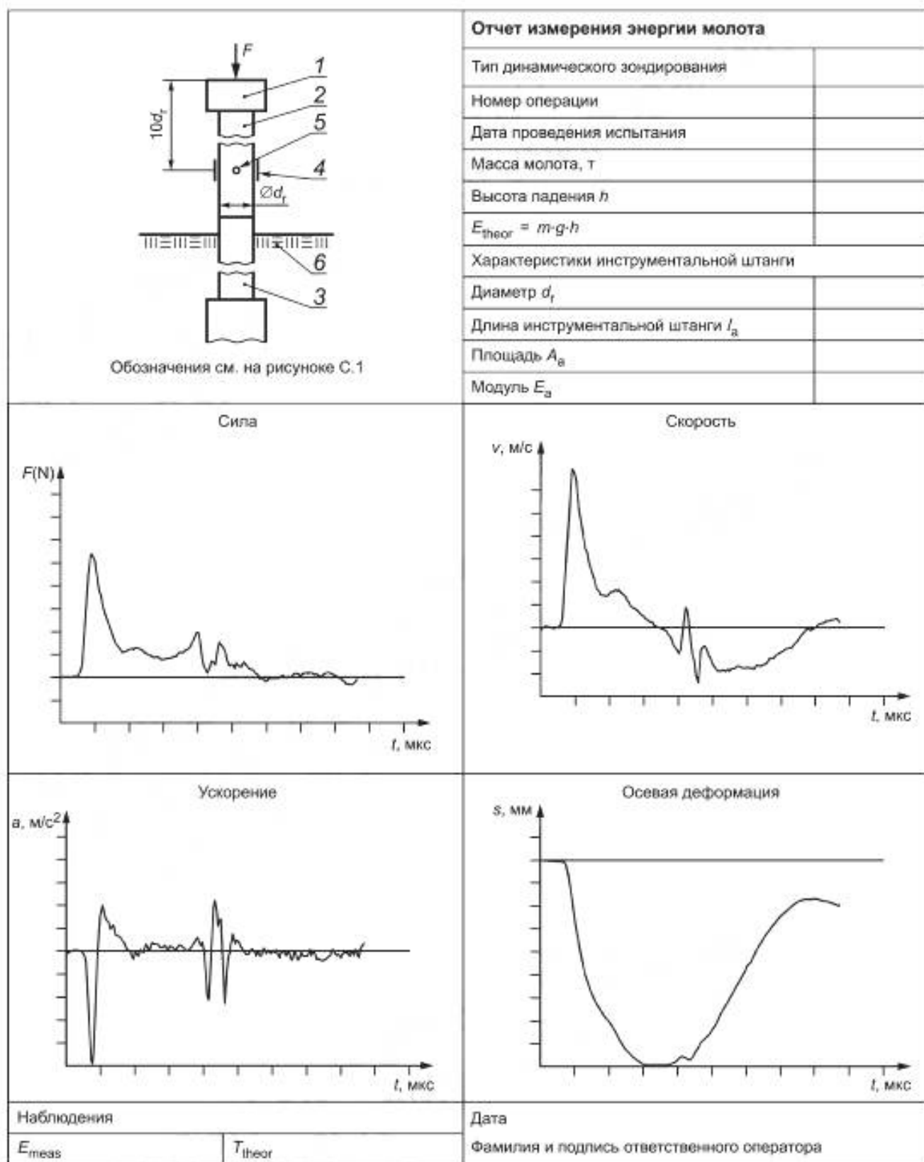
Рисунок С.2 — Пример отчета измерения энергии молота
