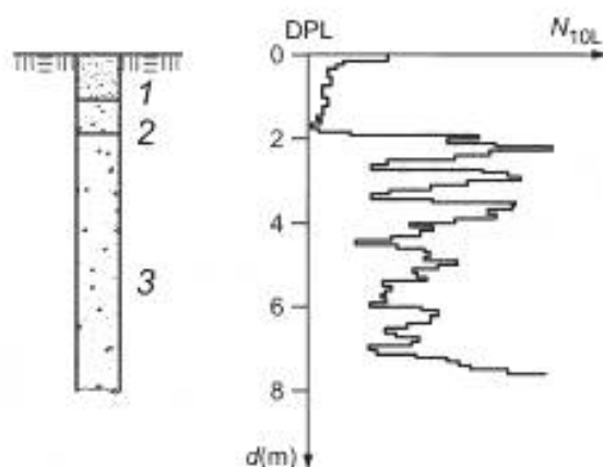
1 — супесь, песчаная; 2 — супесь; 3 — гравий; d — глубина
