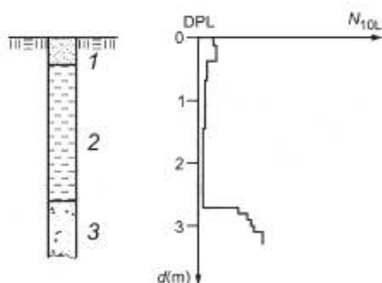
Рисунок D.9 — Динамическое зондирование в разложившемся торфе
