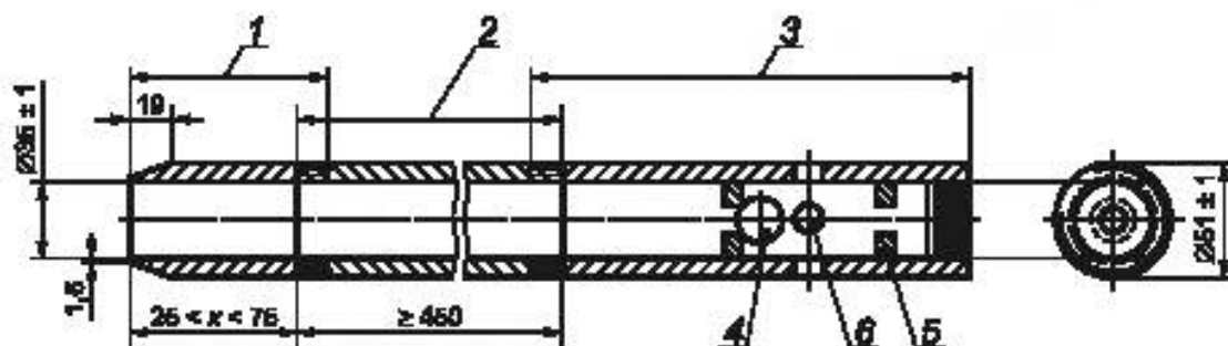
1 — забивной режущий башмак; 2 — разъемный цилиндр; 3 — соединительная муфта; 4 — обратный клапан (рекомендуется: шар диаметром 25 мм и посадочное место для шара диаметром 22 мм); 5 — удерживающие штифты для шара; 6 — четыре отверстия (минимальный диаметр 12 мм); x — длина забивного режущего башмака
