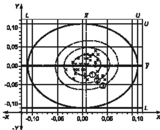
Рисунок 7 — Зона допуска для позиционного допуска
