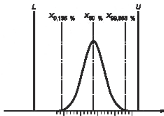
Рисунок 4 — Сопоставление в соответствии с этапом 4
