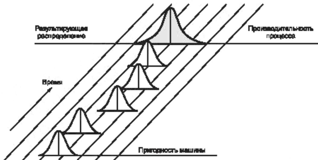
Рисунок 6 — Нестабильный процесс и его пригодность
