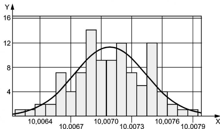
Рисунок 2 — Пример 1 — Гистограмма для нормально распределенных данных
