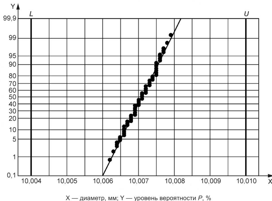
Рисунок 4 — Пример 1 — График вероятности для нормально распределенных данных
