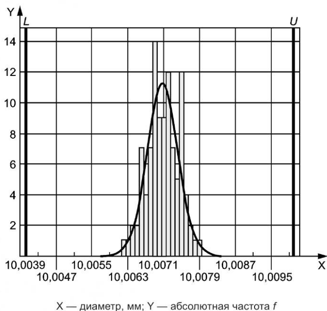
Рисунок 5 — Пример 1 — Анализ пригодности машины для нормально распределенных данных
