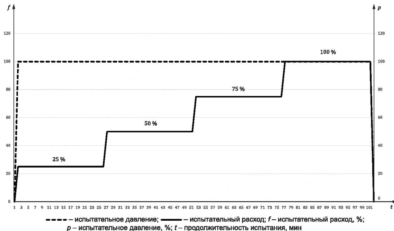
Рисунок 3 — Этапы нагружки
