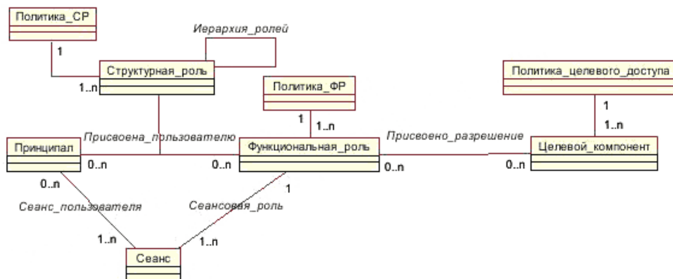
Рисунок 3 – Схема ролевого контроля доступа, управляемого политиками
