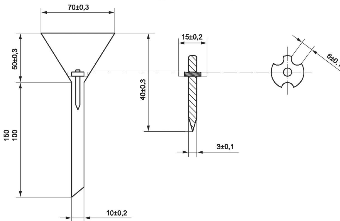
Рисунок 2 — Воронка с зафиксированным металлическим штифтом
