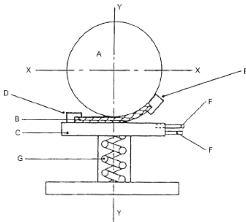
Рисунок 1 — Устройство для измерения адсорбции и десорбции воды
