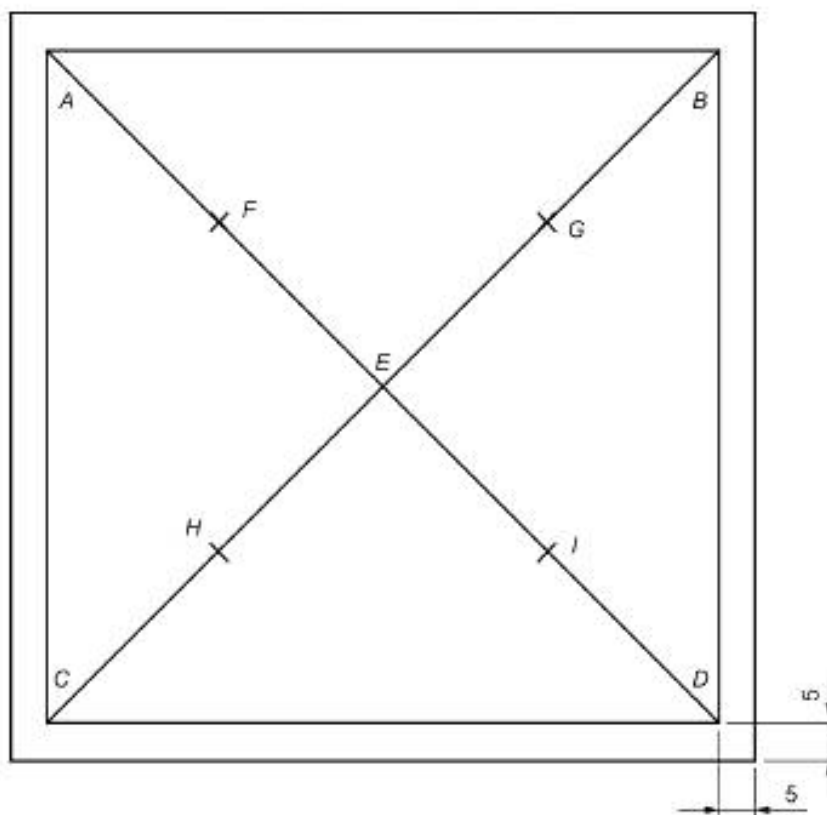
Рисунок 1 — Разметка образца для испытания
