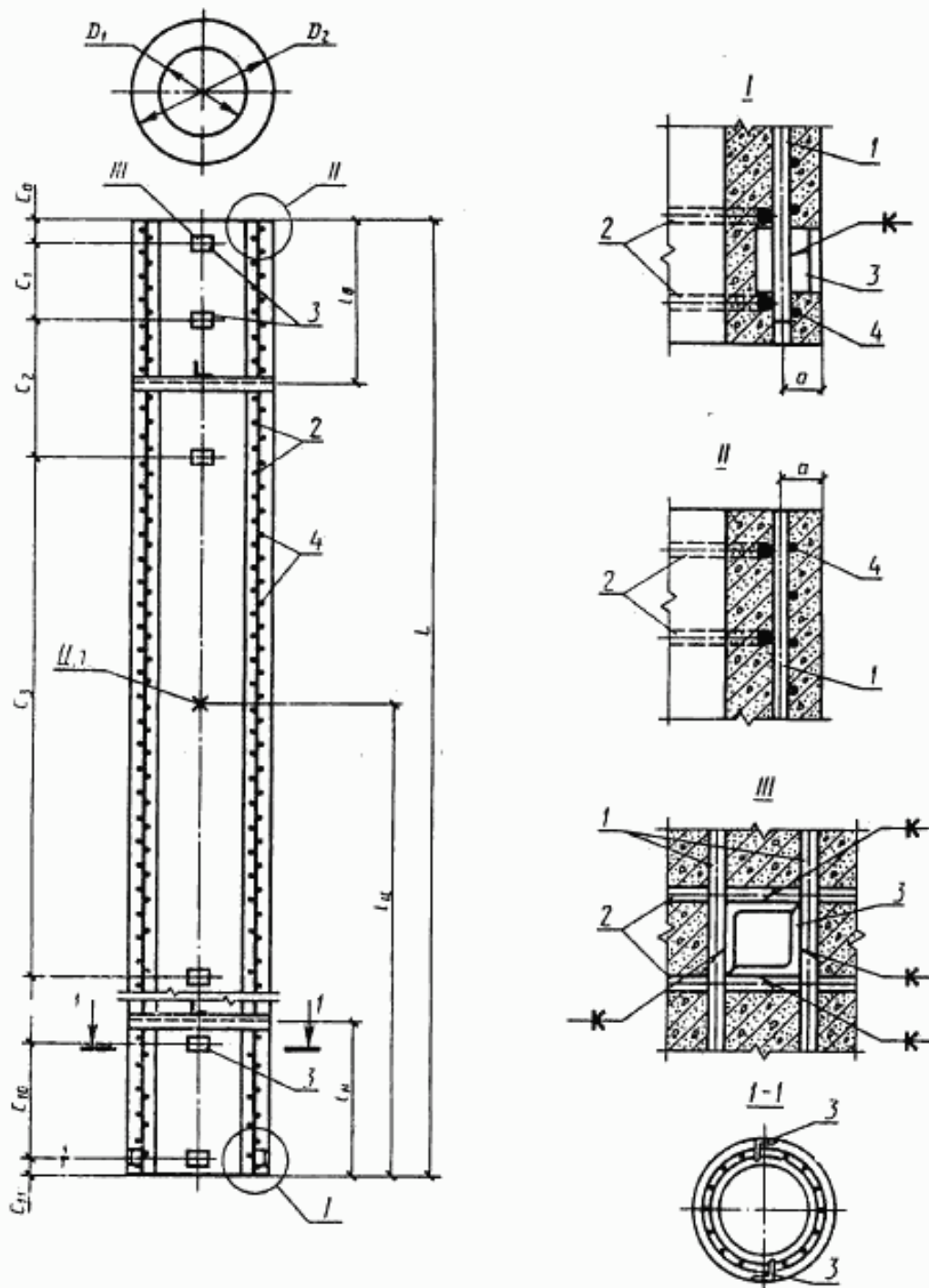
1 — продольная арматура; 2 — монтажные кольца; 3 — закладные изделия; 4 — спираль; a — расстояние от наружной поверхности стойки до оси продольной арматуры; c_1 — c_2 , c_{10} — c_{11} — привязка закладных изделий; c , t — центр тяжести; L — длина стойки; l_{II} — расстояние до центра тяжести; l_{II} , l_{III} — расстояния до мест установки диафрагмы; D_1 — внутренний диаметр стойки; D_2 — наружный диаметр стойки
