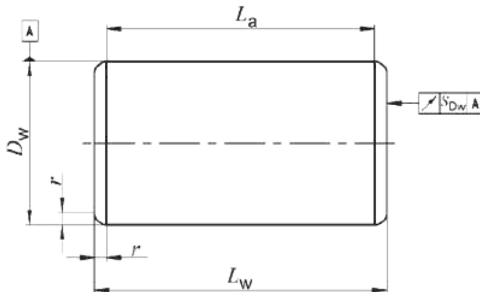
Рисунок 1 – Цилиндрический ролик
