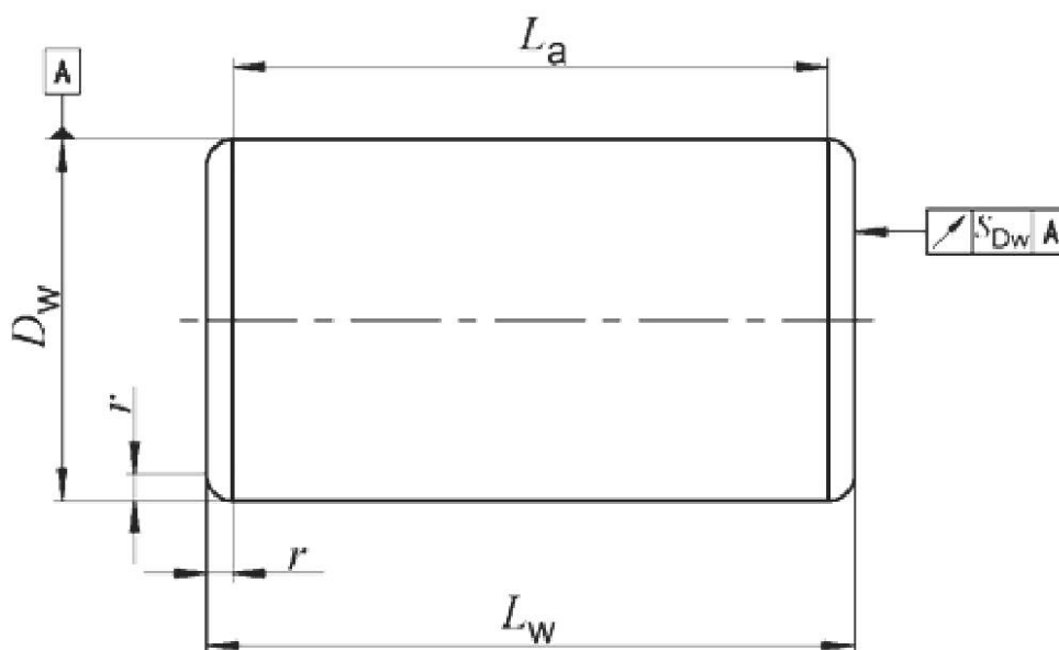
Рисунок 1 – Цилиндрический ролик
