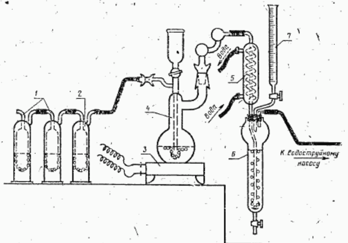
1—склянки-ловушки, заполненные серной кислотой; 2—склянка-ловушка, заполненная водой; 3—электролитка; 4—дистилляционная колба из термостойкого стекла вместимостью 500 мл с притертой пробкой, снабженной капельной воронкой с краном; 5—холодильник; 6—сосуд для улавливания аммиака; 7—микробюретка 2-го класса
