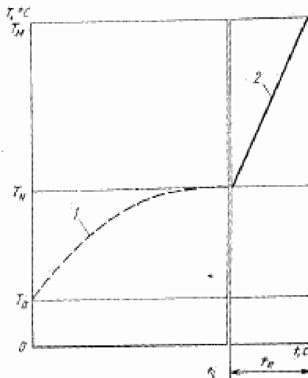
График определения времени нагрева t_w
