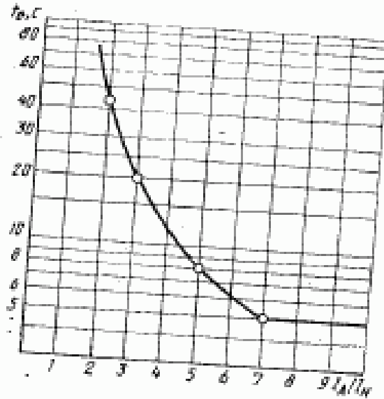
График определения минимального значения времени нагрева t_0
