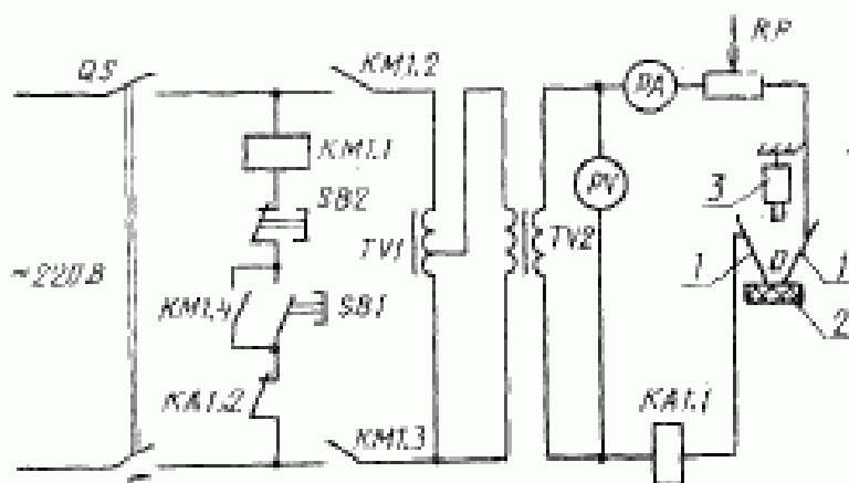
Принципиальная электрическая схема установки испытаний на трекингостойкость
