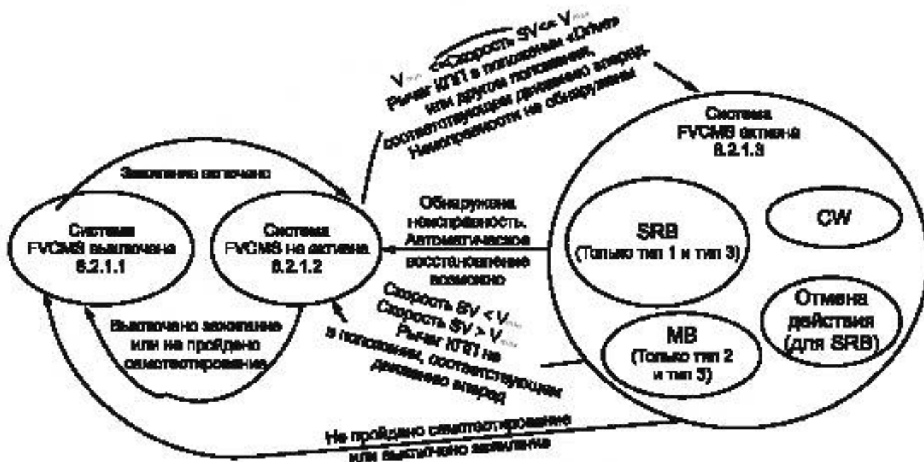
Рисунок 2 — Диаграмма состояний и переходов системы FVCMS
