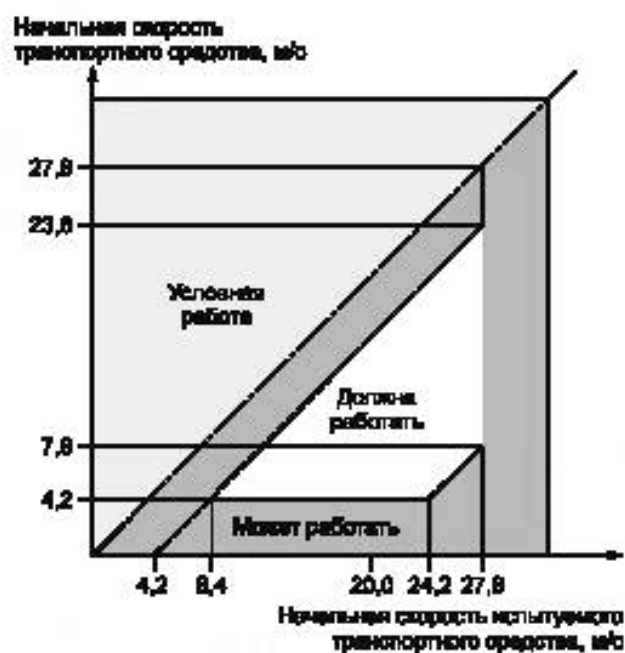
Рисунок 4 — Границы рабочих диапазонов скоростей системы FVCMS
