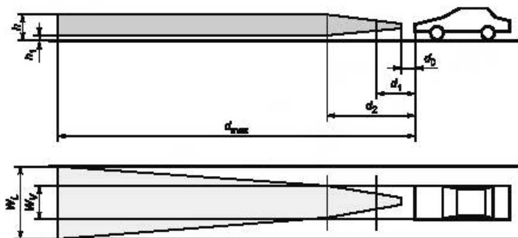
Рисунок 5 — Минимальная зона обнаружения
