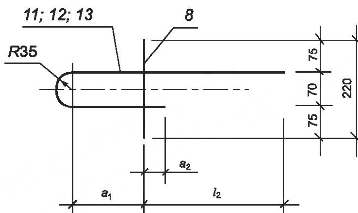
Рисунок Б.8 — Каркасы КР6—КР8
