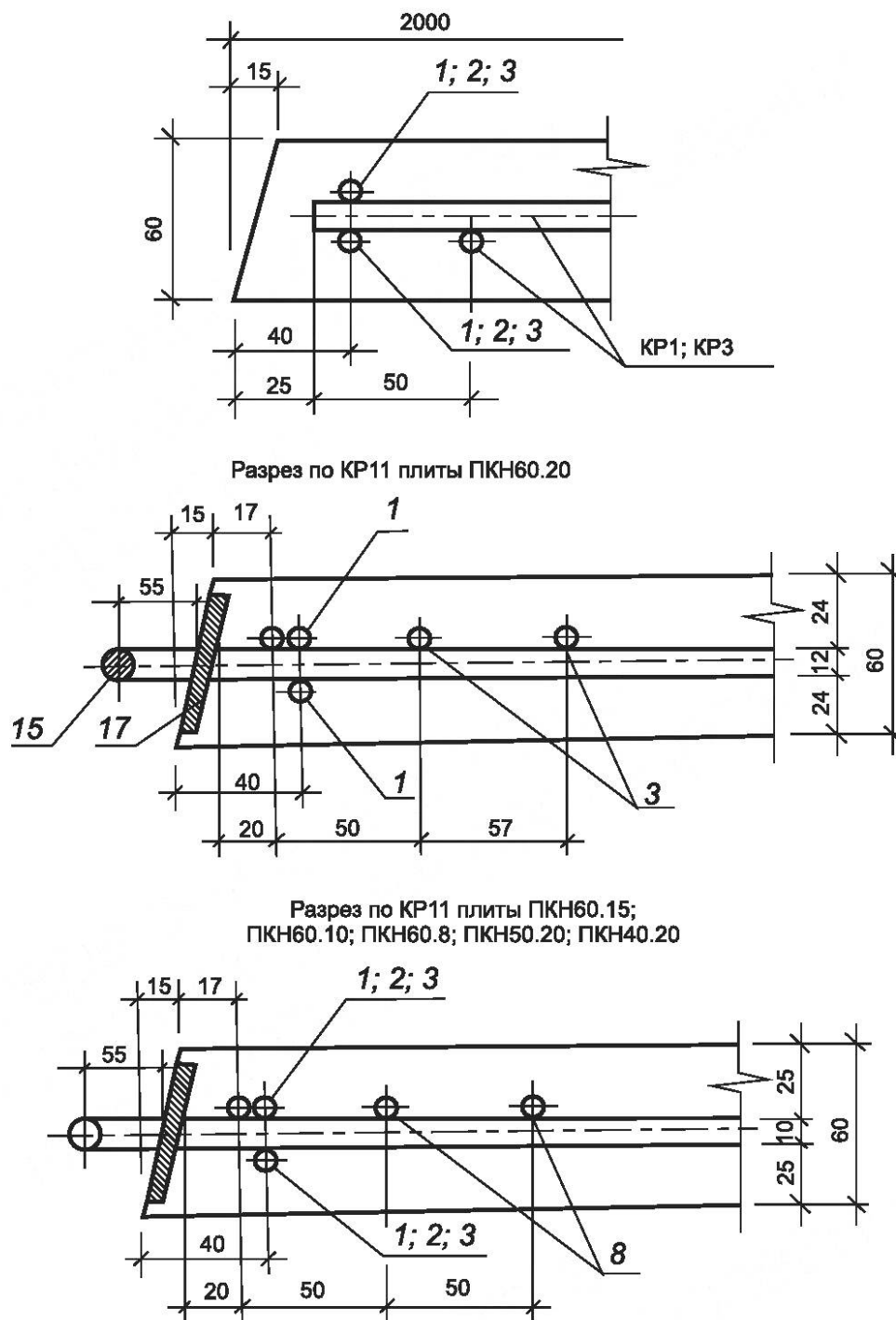
Рисунок Б.4 — Схемы армирования плит. Узел 1. Разрезы по каркасу КР11
