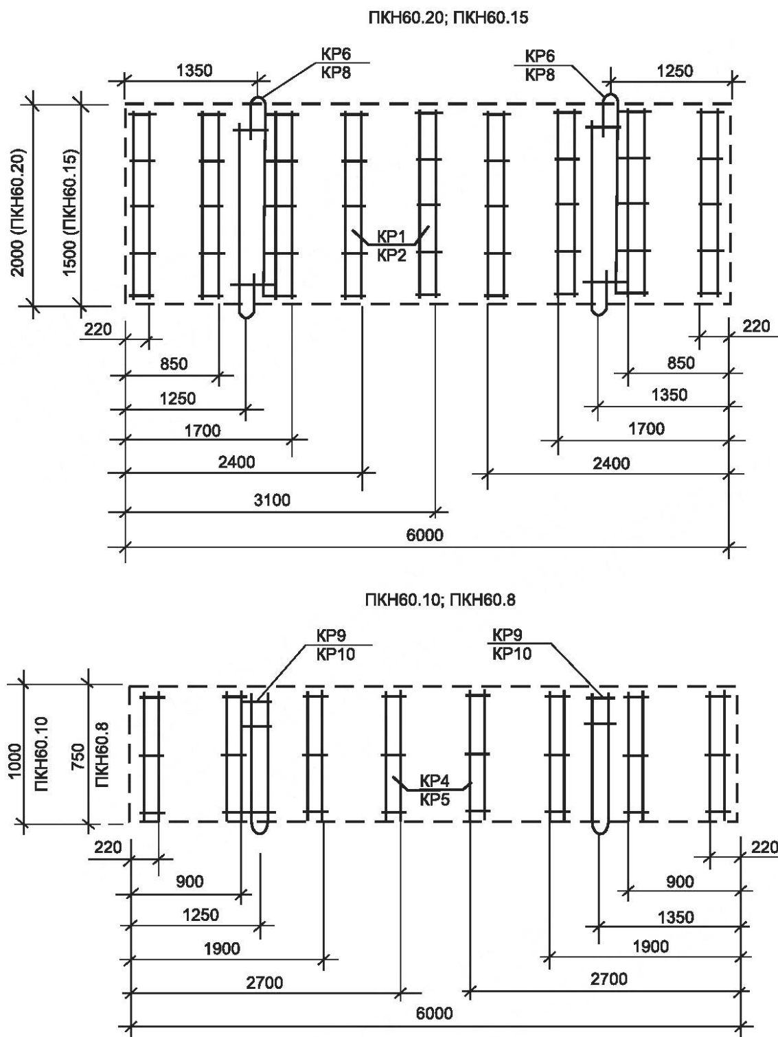
Рисунок Б.5 — Схемы расположения каркасов плит ПКН60.20, ПКН60.15, ПКН60.10 и ПКН60.8
