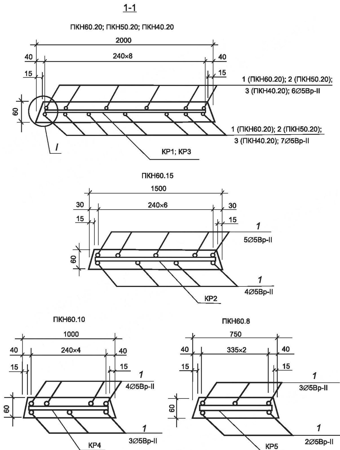
Рисунок Б.3 — Схемы армирования плит. Сечения 1-1
