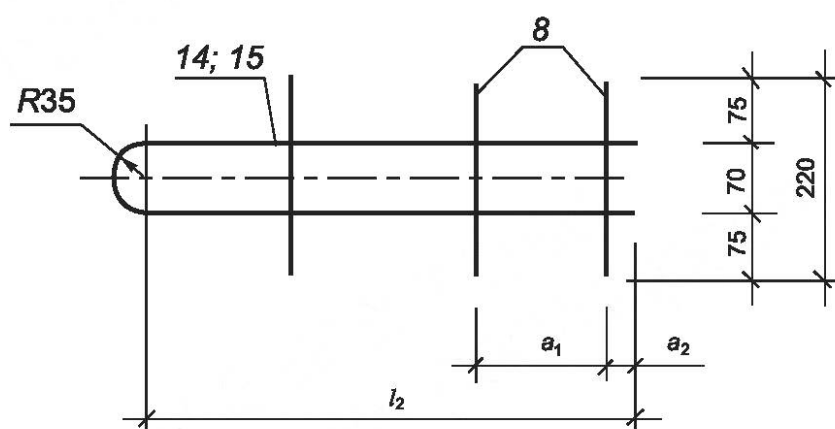
Рисунок Б.9 — Каркасы КР9, КР10
