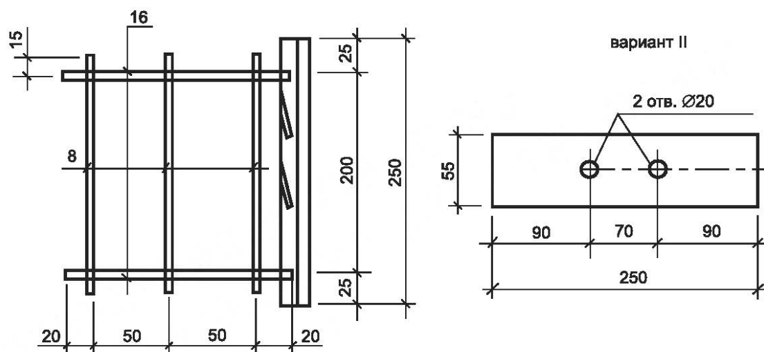
Рисунок Б.10, лист 2
