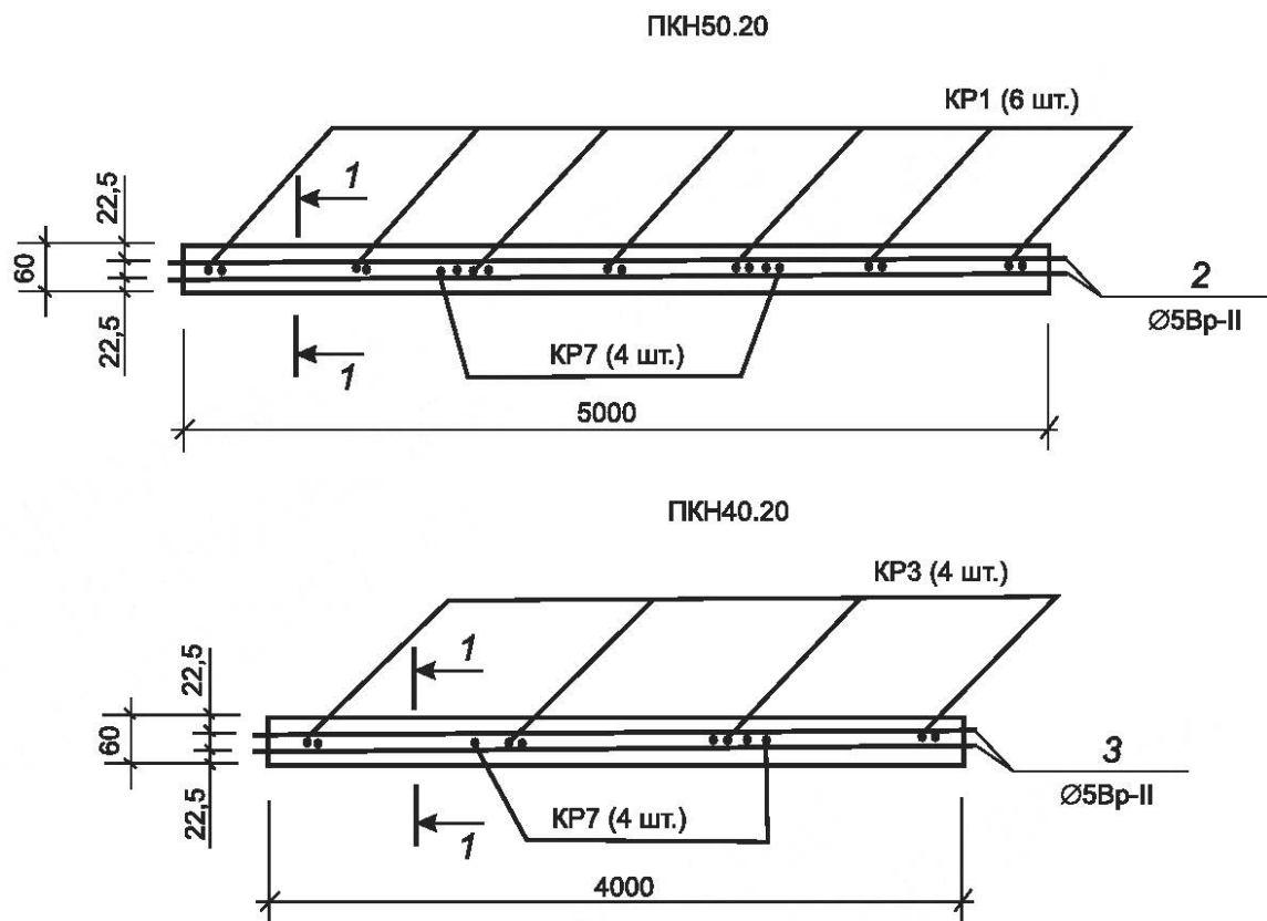
Рисунок Б.2 — Схемы армирования плит ПКН50.20 и ПКН40.20
