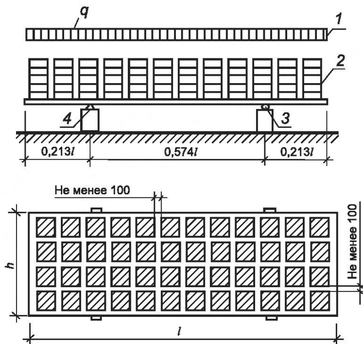
1 — теоретическая схема нагрузки; 2 — нагрузка; 3 — подвижная опора; 4 — неподвижная опора
