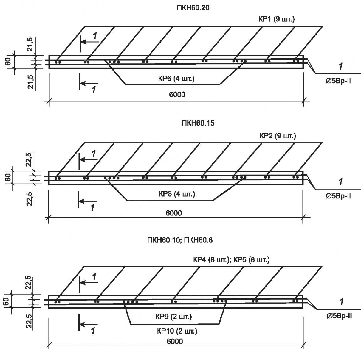
Рисунок Б.1 — Схемы армирования плит ПКН60.20, ПКН60.15, ПКН60.10 и ПКН60.8
