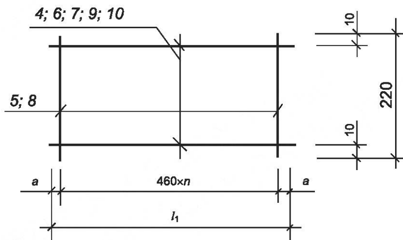
Рисунок Б.7 — Каркасы КР1—КР5
