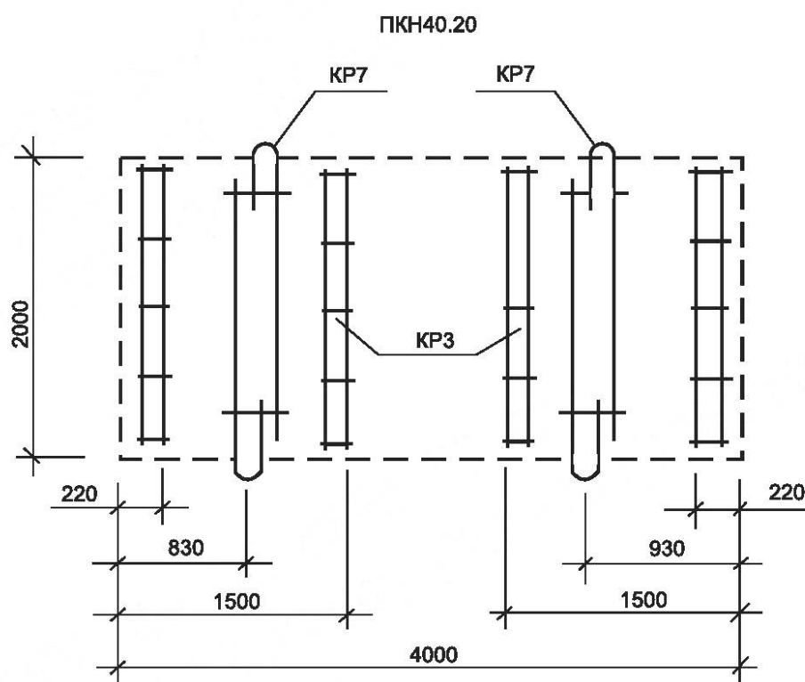
Рисунок Б.6 — Схемы расположения каркасов плит ПКН50.20, ПКН40.20
