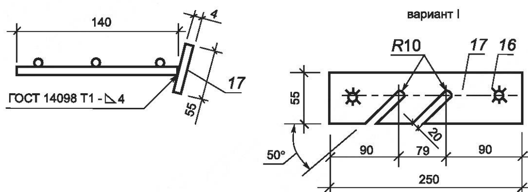
Рисунок Б.10, лист 1 — Каркас КР11. Допускается применение полосы 17 толщиной 5 мм и изменение ее ширины в пределах \pm 5 мм
