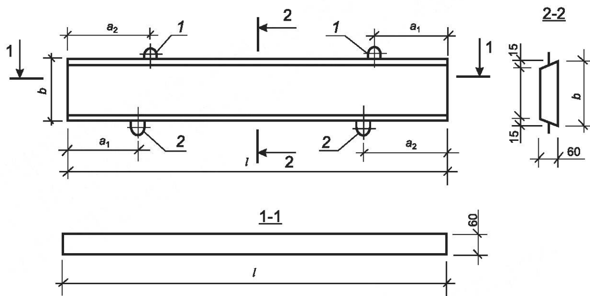
Рисунок А.1 — Плита ПКН (только для плит при b = 750 и 1000 мм)
