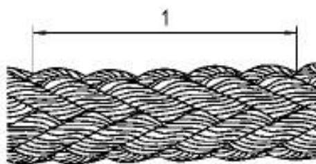
Рисунок 5 Шаг плетения для 8-прядного плетеного каната
