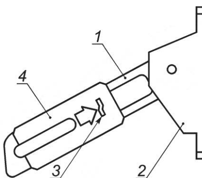
1 — поворотная пластина; 2 — основание; 3 — замочная скважина замка безопасности; 4 — подвижная плата с замком
