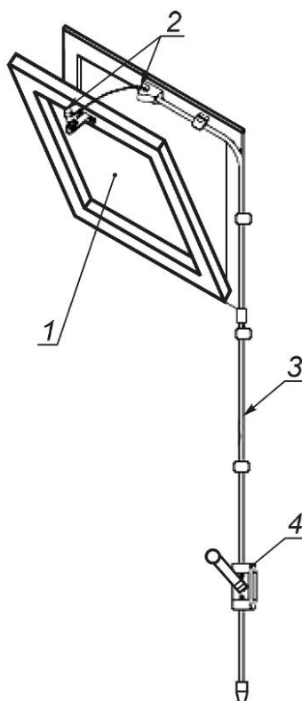
Рисунок Б.12 — Фрамужный механизм с применением механических рычагов управления
