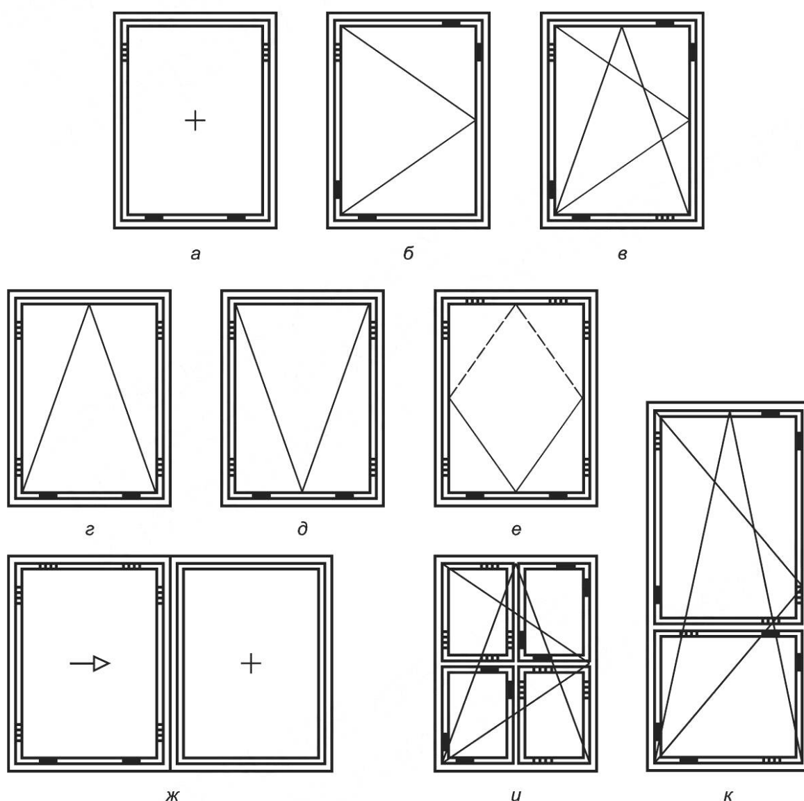
а — неоткрывающийся оконный блок; б — оконный блок с поворотной (распашной) створкой; в — оконный блок с поворотно-откидной створкой; г — оконный блок с откидной створкой; д — оконный блок с подвесной створкой; е — оконный блок со среднеподвесной створкой; ж — оконный блок с раздвижной створкой; и, к — оконные блоки со створками сложной конструкции; ■ — несущая подкладка; ▤ — дистанционная подкладка
