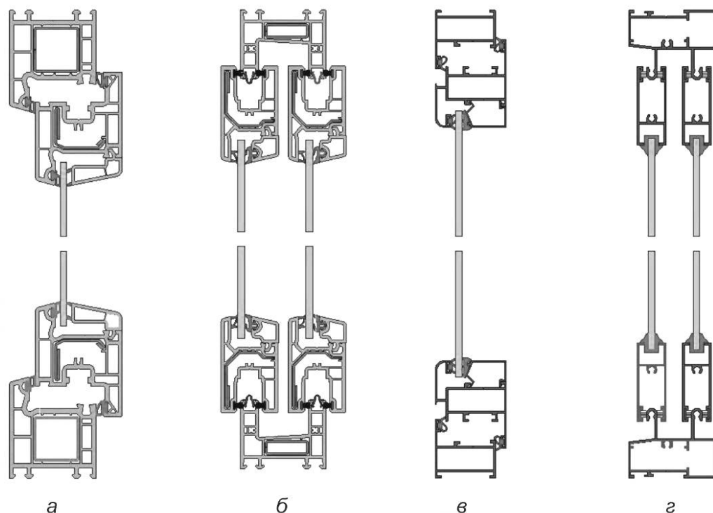
а — блок остекления балкона из ПВХ-профиля с поворотным (поворотн-откидным) открыванием створок; б — блок остекления балкона из ПВХ-профиля с параллельно-раздвижным открыванием створок; в — блок остекления балкона из алюминиевого профиля с поворотным (поворотн-откидным) открыванием створок; г — блок остекления балкона из алюминиевого профиля с параллельно-раздвижным открыванием створок
