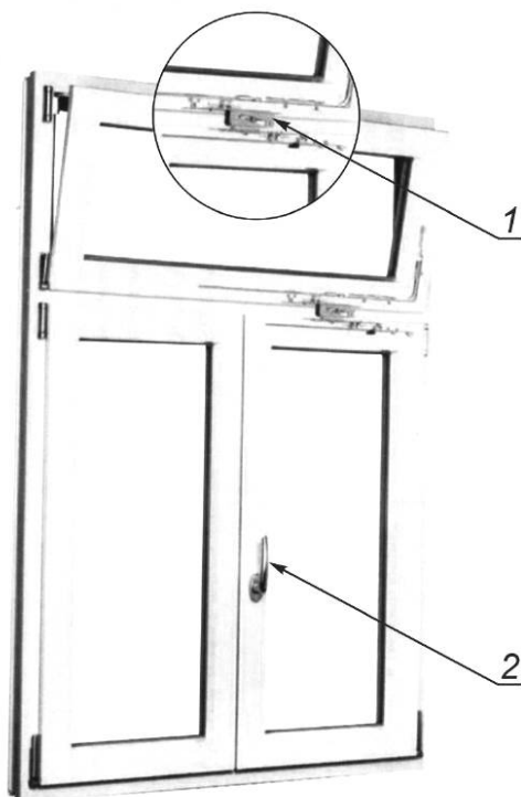
Рисунок Б.13 — Пример установки фрамужного механизма открывания, работающего от центральной ручки
