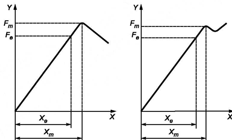
Рисунок 2 — Пример кривой «нагрузка — перемещение» для режима В
