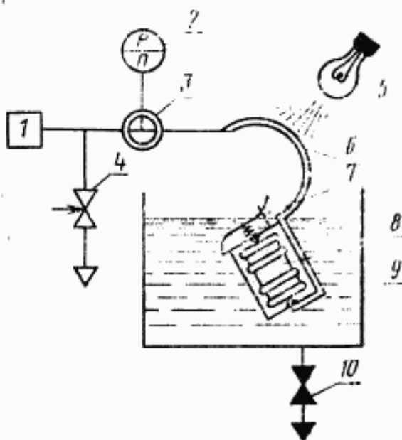
Схема установки для испытания фильтрующе-поглощающих коробок противогазов
