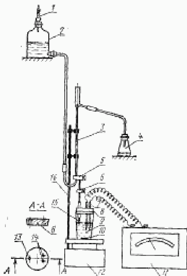
Общий вид потенциометрической установки
