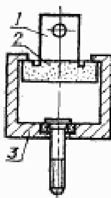
1—испытательная головка; 2—образец; 3—захват.
