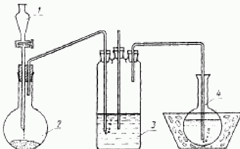
Прибор для получения хлора
