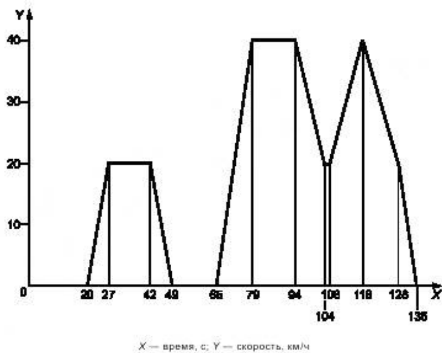
Рисунок А.1 — Десятирежимный ездовой цикл
