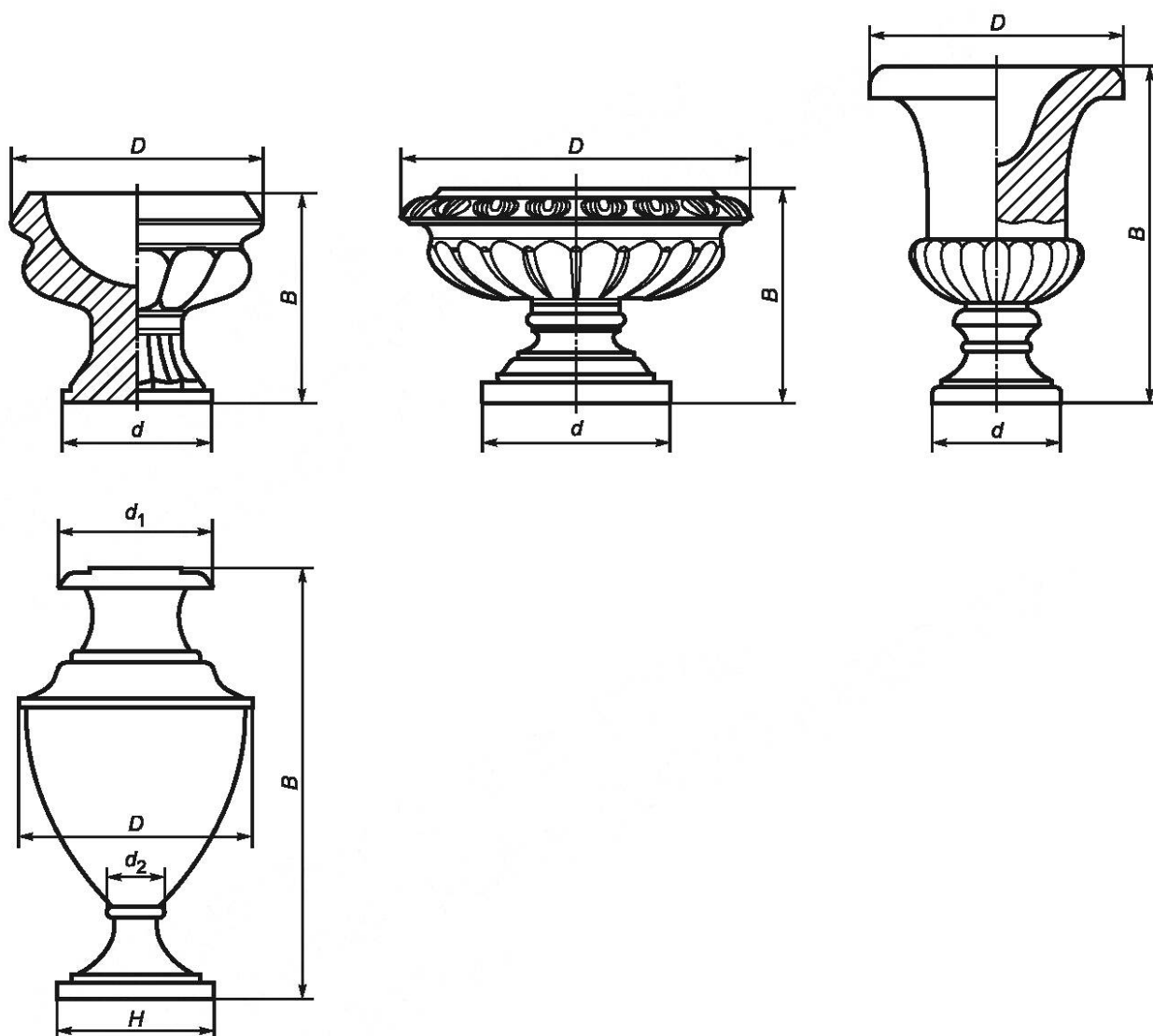
Рисунок 12 — Вазы
