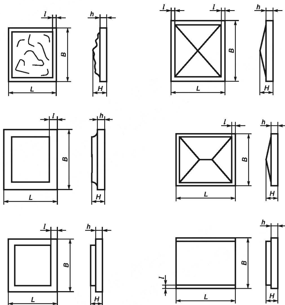
Рисунок 1 — Рустовые камни
