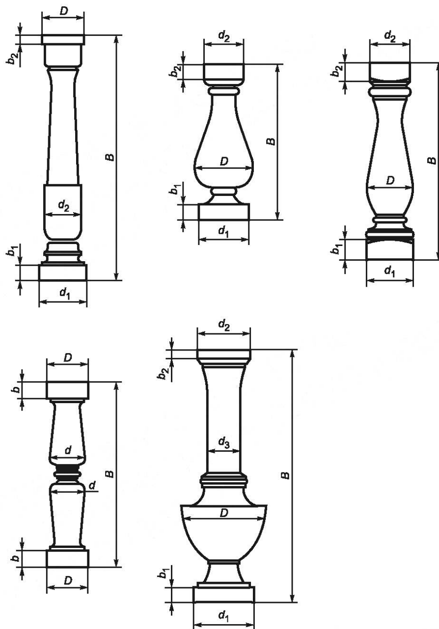
Рисунок 11 — Балясины
