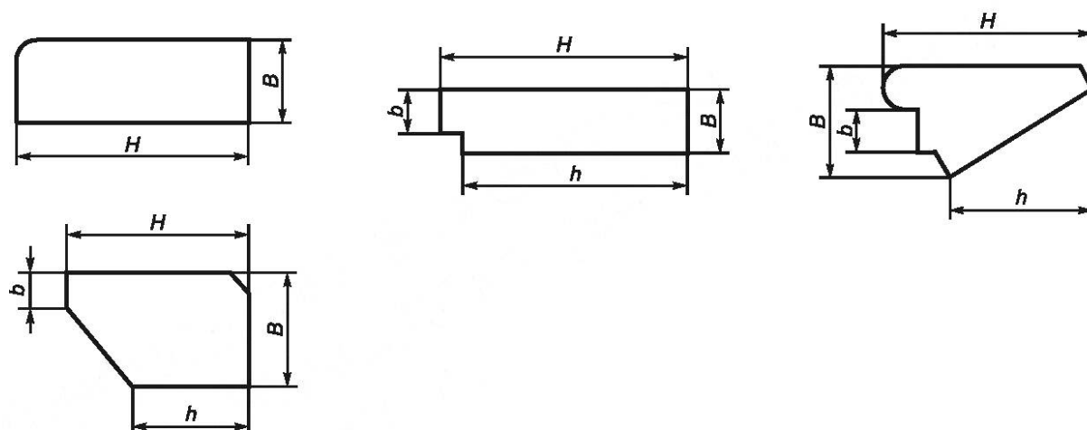
Рисунок 5 — Цельные ступени
