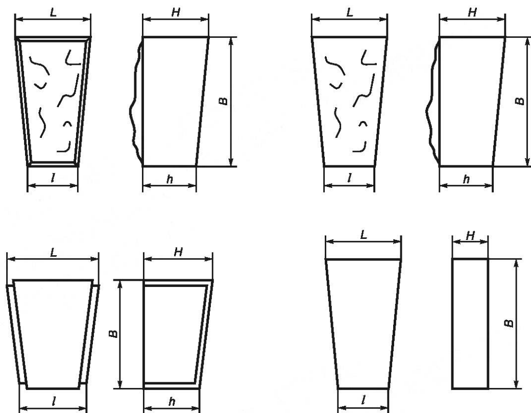
Рисунок 2 — Замковые камни
