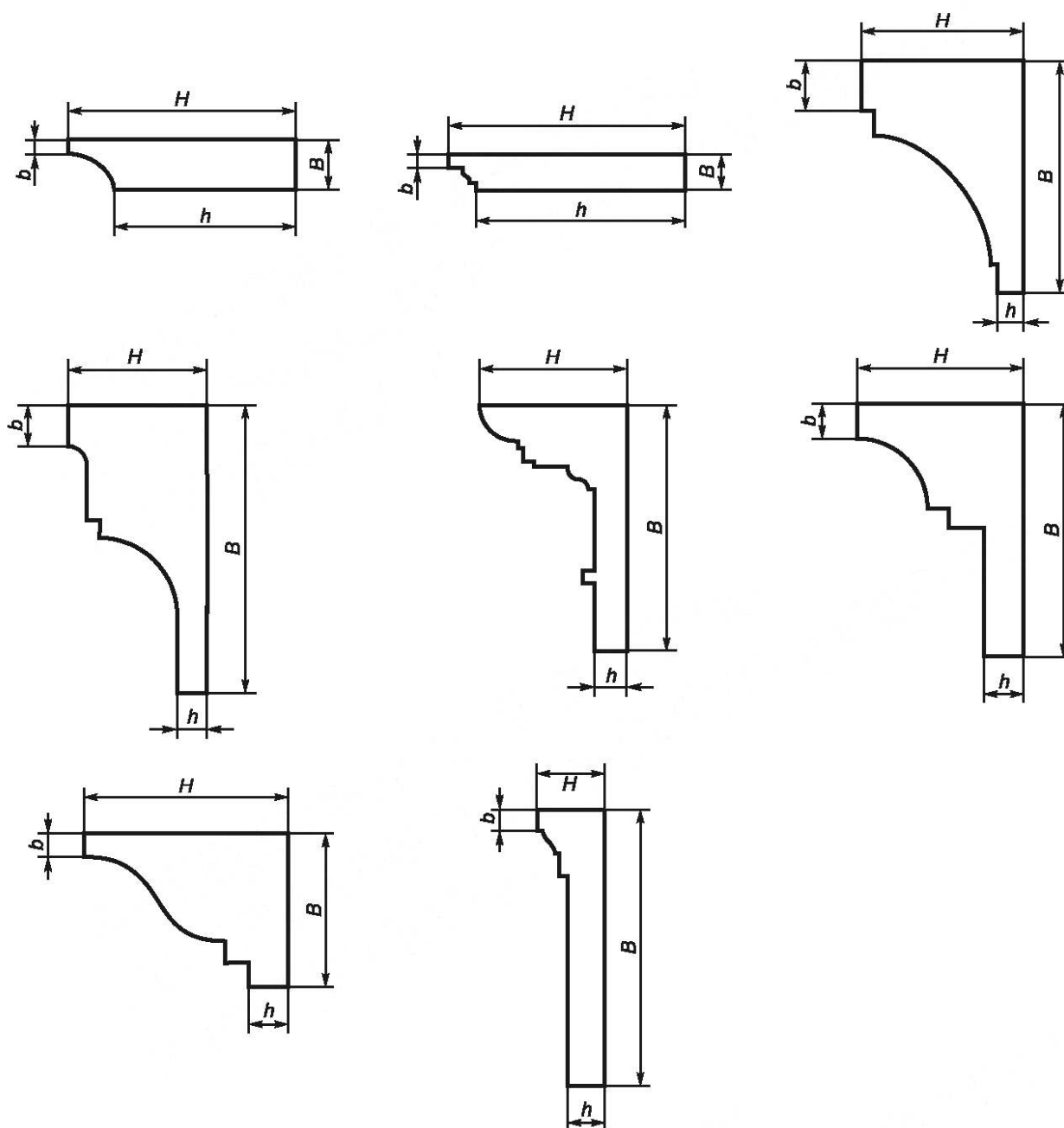
Рисунок 3 — Карнизы
