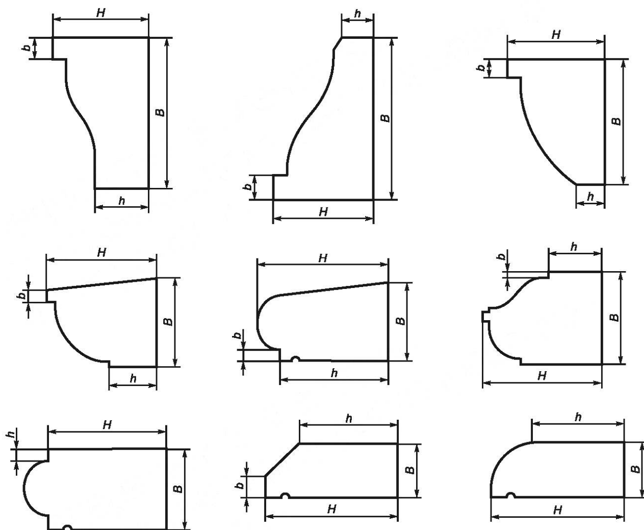
Рисунок 4 — Кордонные камни
