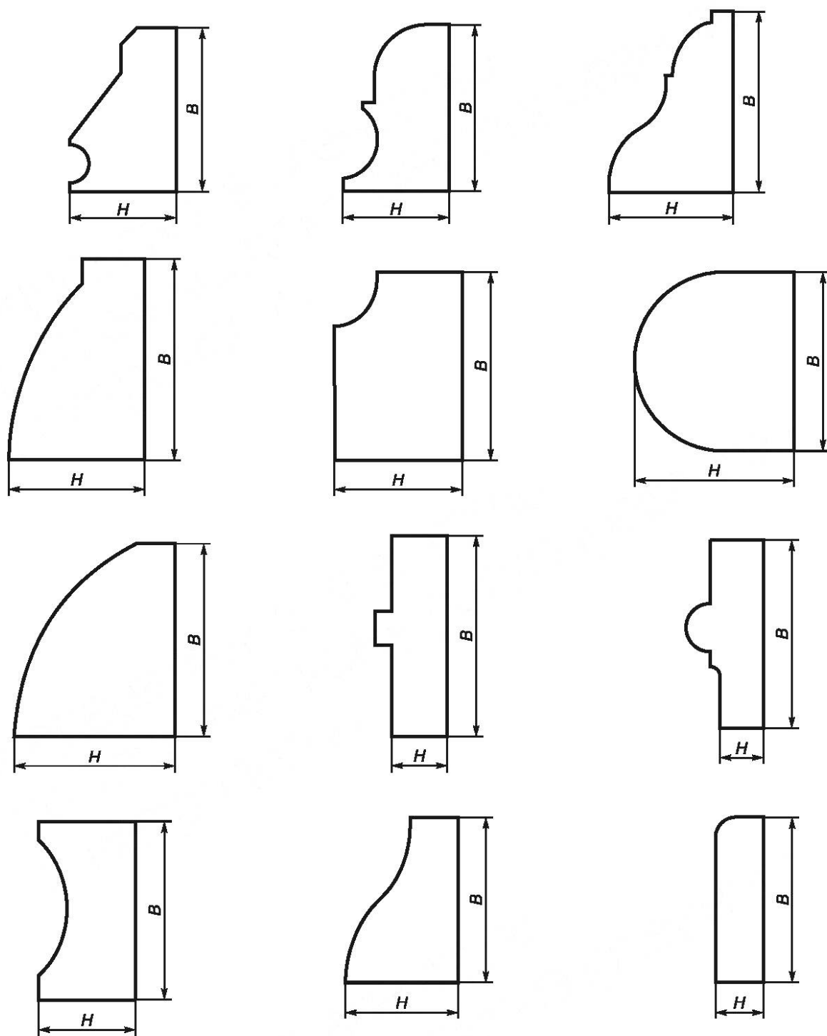
Рисунок 7 — Напольные плинтусы
