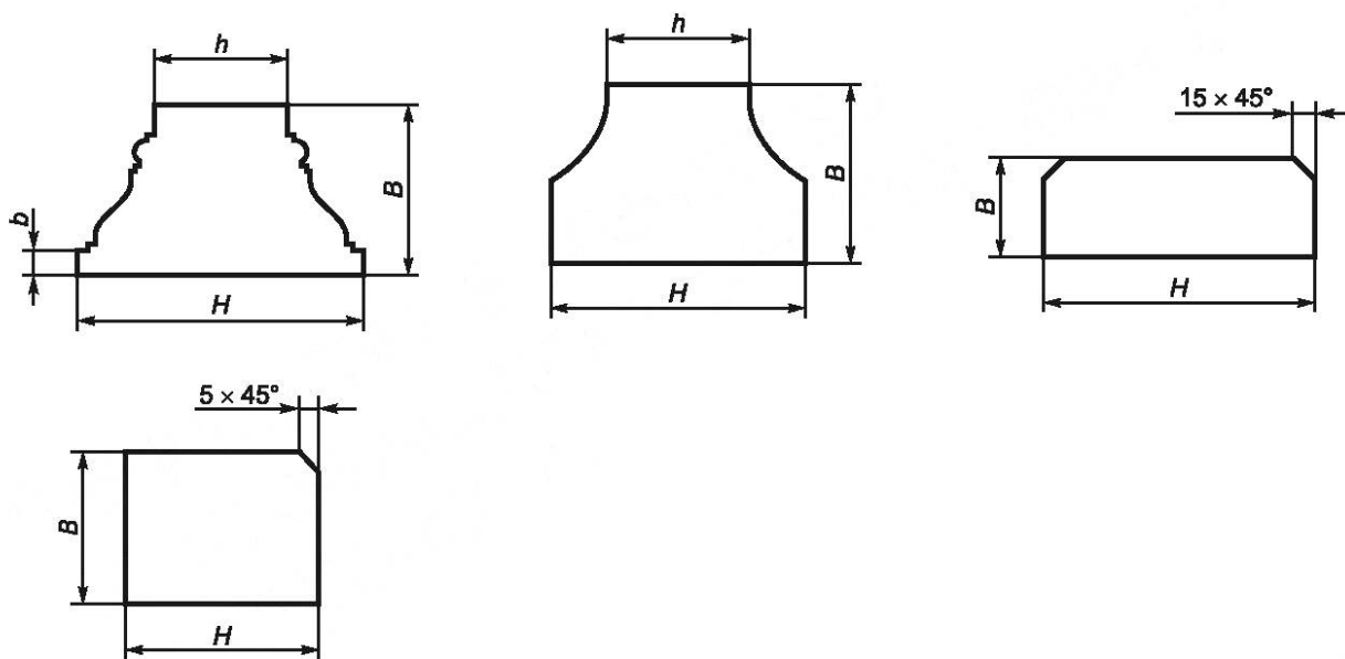
Рисунок 8 — Основания балюстрад
