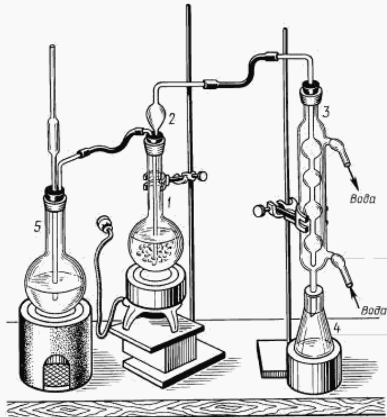
Прибор для отгонки летучих кислот
