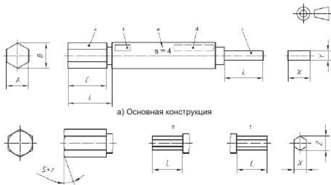
а) Основная конструкция б) Дополнения к конструкции GO калибра или NOT GO калибра для малых размеров
