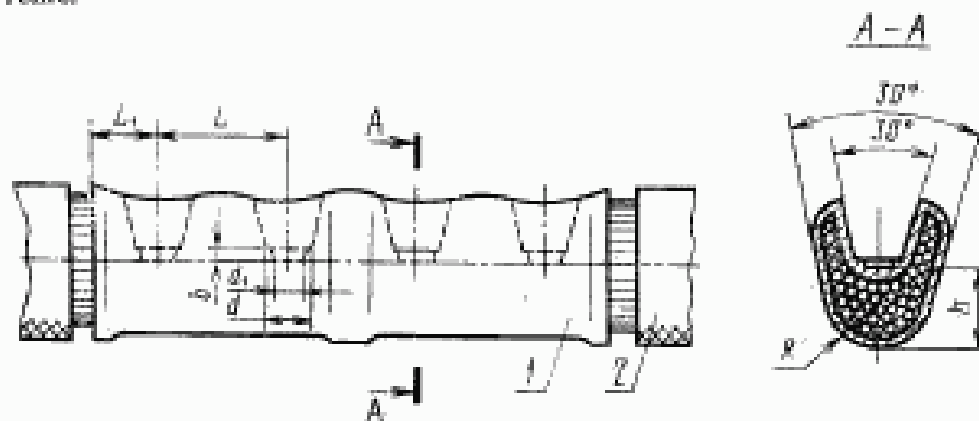
1—гильза; 2—кабель. Размеры в мм
