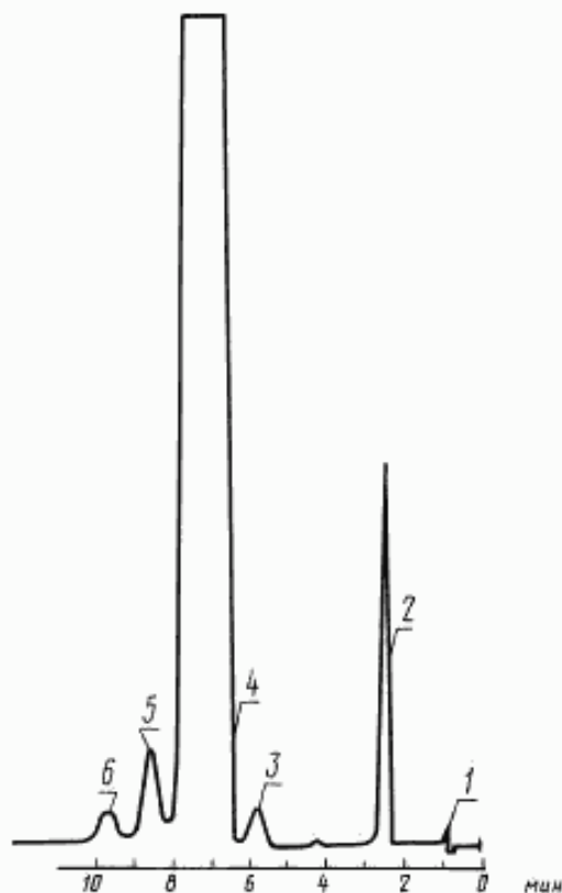
Типовая хроматограмма
