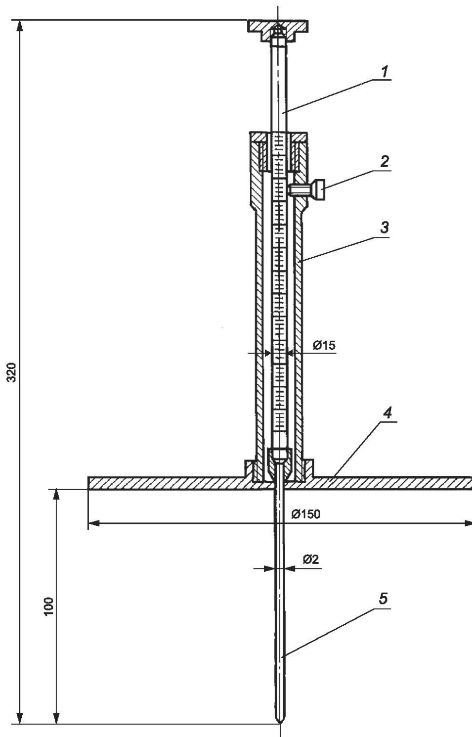
Рисунок 1 — Схема толщиномера
