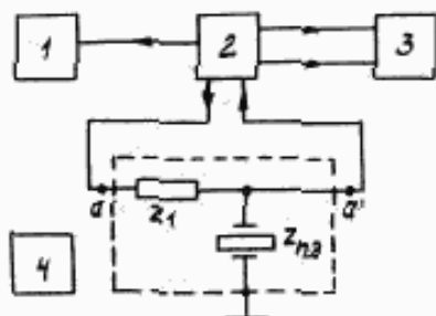
1 — частотомер; 2 — измеритель АЧХ; 3 — графопостроитель; Z_{н.з} — проверяемый ПЭП; Z_1 — электрическая нагрузка; 4 — акустическая нагрузка
