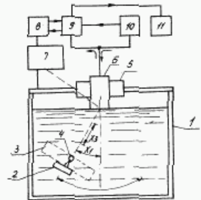
1 — иммерсионная ванна; 2 — узел фиксации отражателя; 3 — плоский отражатель; 4 — сферический отражатель; 5 — узел фиксации ПЭП; 6 — проверяемый ПЭП; 7 — механизм перемещения по координатам X_1 , X_3 ; 8 — графопостроитель; 9 — приемник; 10 — генератор; 11 — осциллограф
