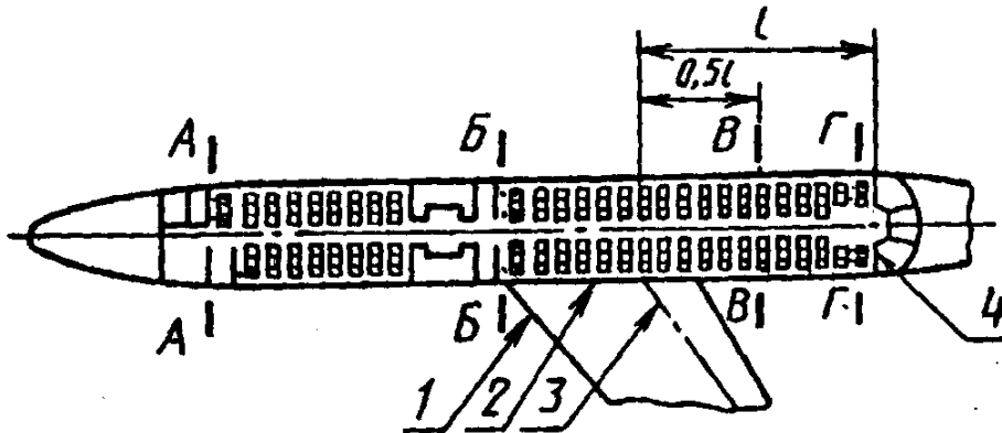
А, Б, В, Г — сечения; 1 — передняя кромка крыла; 2 — корневая нервюра; 3 — задний лонжерон; 4 — задняя стенка пассажирской кабины Черт. 6
