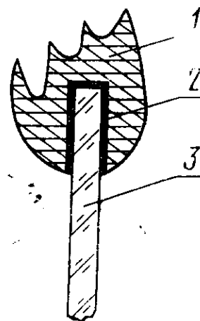
1—резиновый уплотнитель; 2—мастика; 3—стекло
