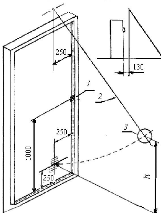
Рисунок В.3 – Схема проведения испытания на сопротивление удару мягким не упругим телом (грузом) в направлении закрывания дверного полотна
