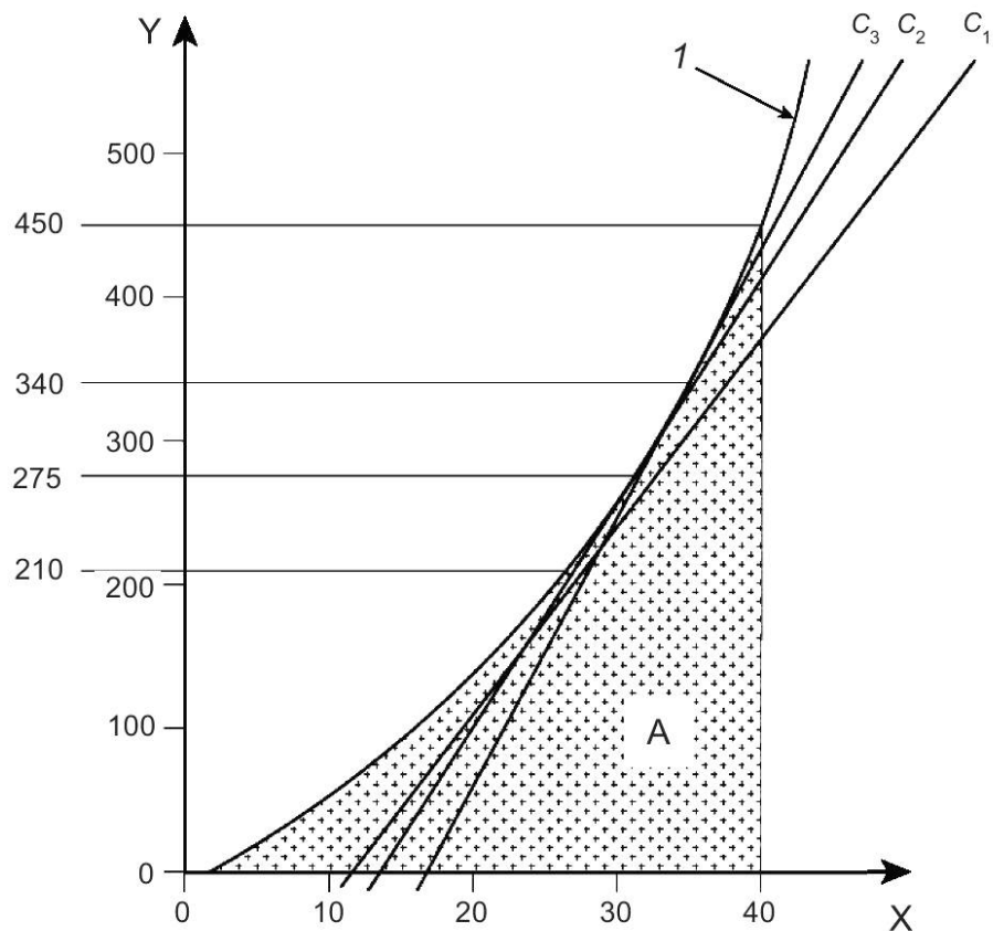
Рисунок 4 — Определение показателя жесткости
