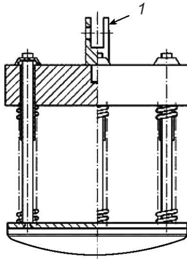
1 — шарнир подъемного устройства, не препятствующий свободному падению
