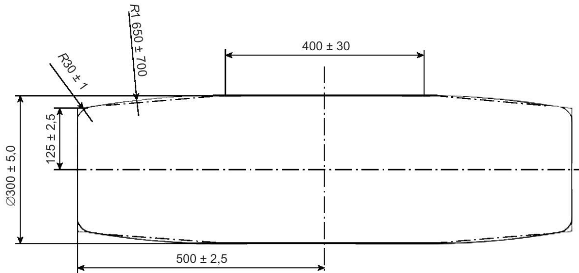
Рисунок 3 — Ролик
