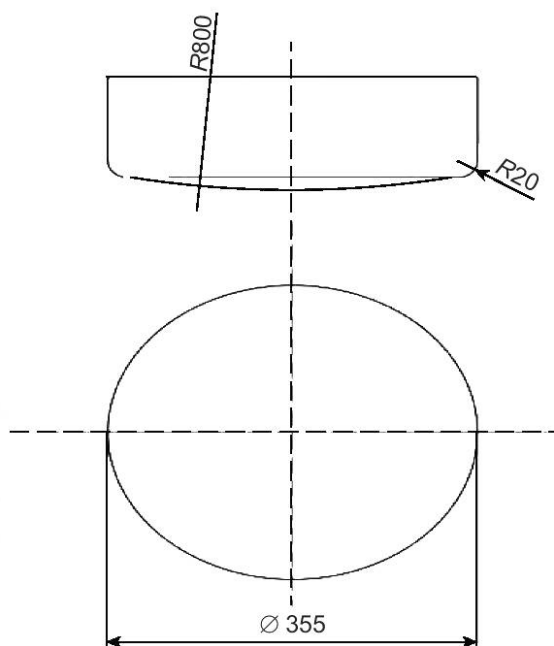
Рисунок 2 — Нагрузочная площадка
