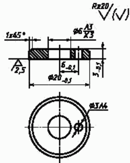
Рисунок Б.3 — Шайба
