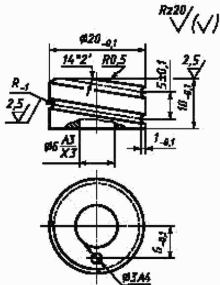
Рисунок Б.2 — «Улитка»
