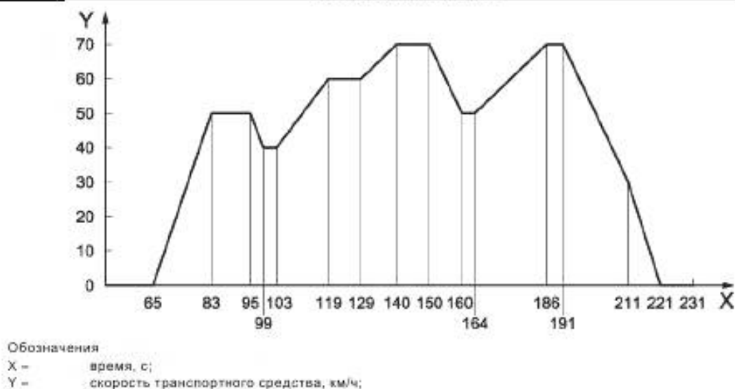
Рисунок А.2 — Последовательность испытаний транспортного средства по 15 режимному циклу
