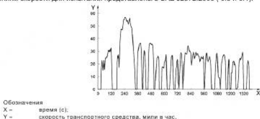
Рисунок С.1 — Последовательность испытаний транспортного средства, имитирующих городское движение в условиях США, в соответствии с городским динамометрическим циклом движения (UDDS)
