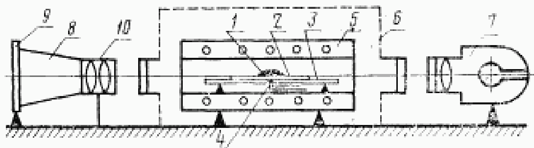
Схема установки для проведения испытаний
