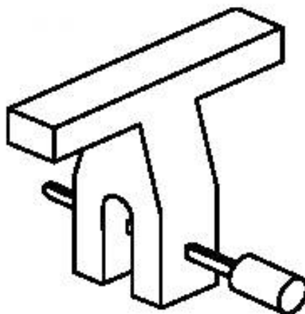
Рисунок 1 — Держатель образца с сердечником
