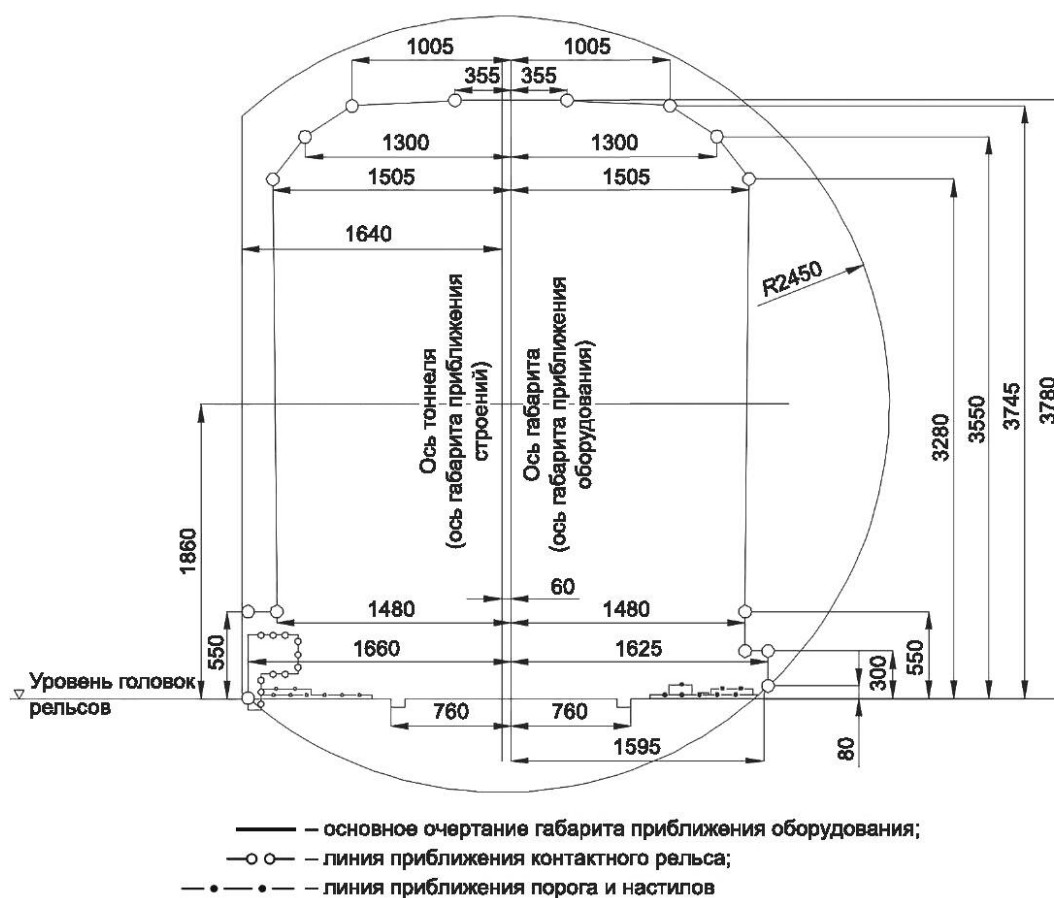
Рисунок 15 — Совмещенные габариты приближения строений C_{мз} и приближения оборудования O_{мз} для станций закрытого типа
