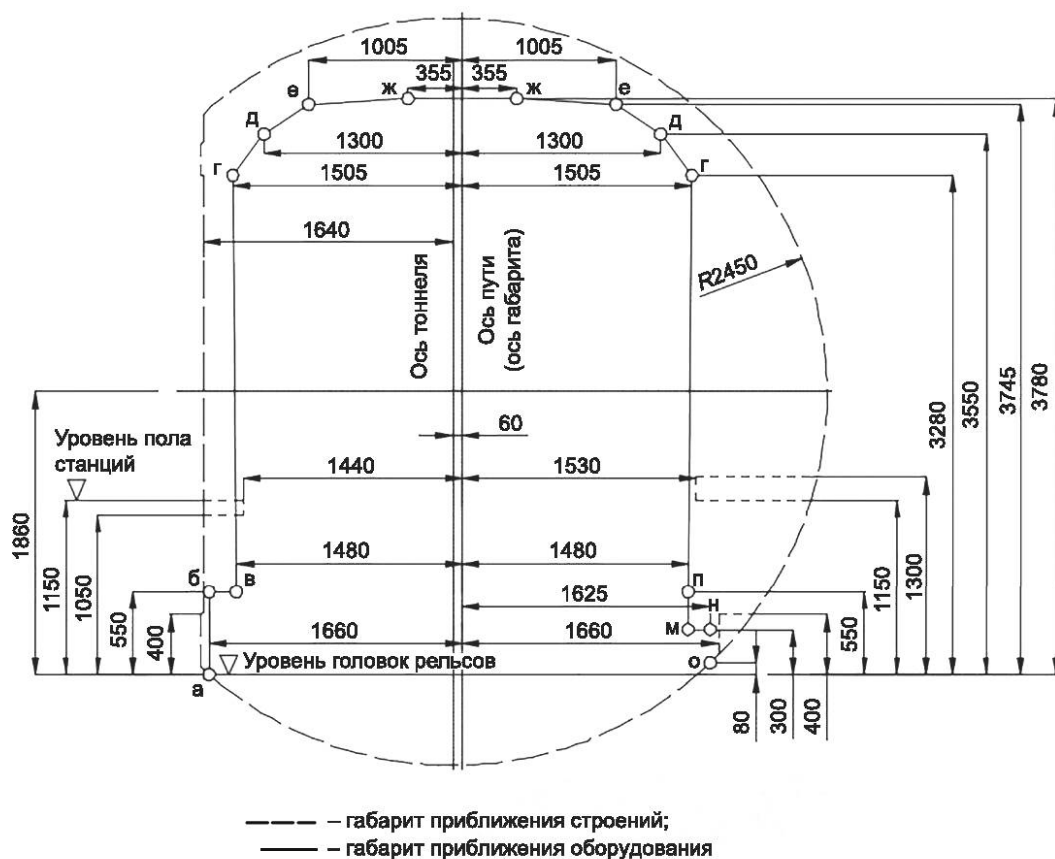
Рисунок 8 — Габариты приближения строений C_{мз} и приближения оборудования O_{мз} станций закрытого типа
