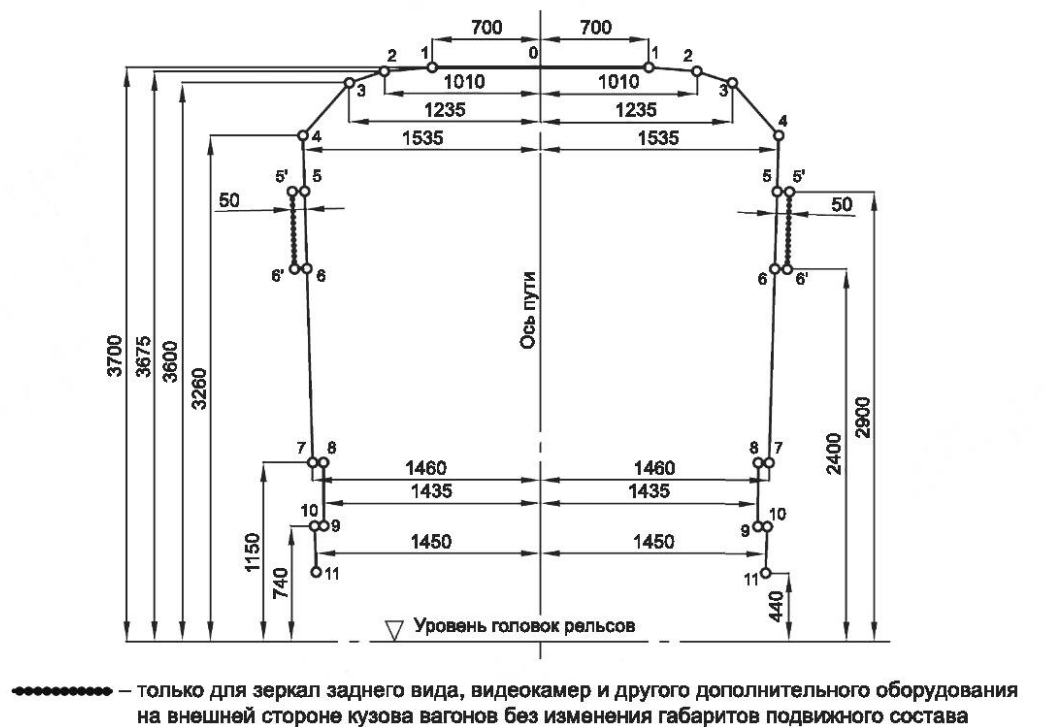
Рисунок 10 — Габарит М. Верхнее очертание габарита М
