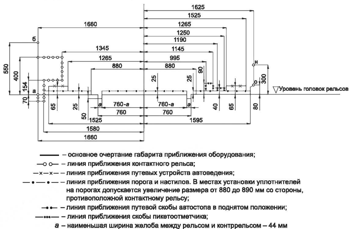
Рисунок 9 — Нижнее очертание габарита приближения оборудования O_{мз} станций закрытого типа
