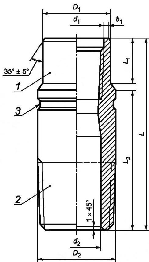
1 — муфтовый конец; 2 — nippleный конец; 3 — маркировочный пояс
