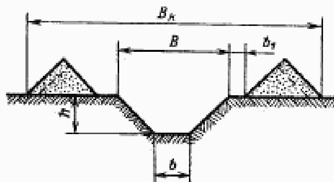
h —глубина канала; b —ширина канала по дну; B —ширина канала по верху; B_k —ширина основания канальера (ширина разбрасывания); b_1 —ширина бермы
