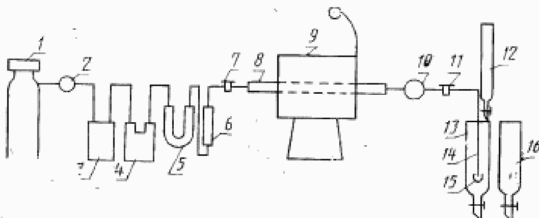
Схема установки для определения серы титриметрическим методом
