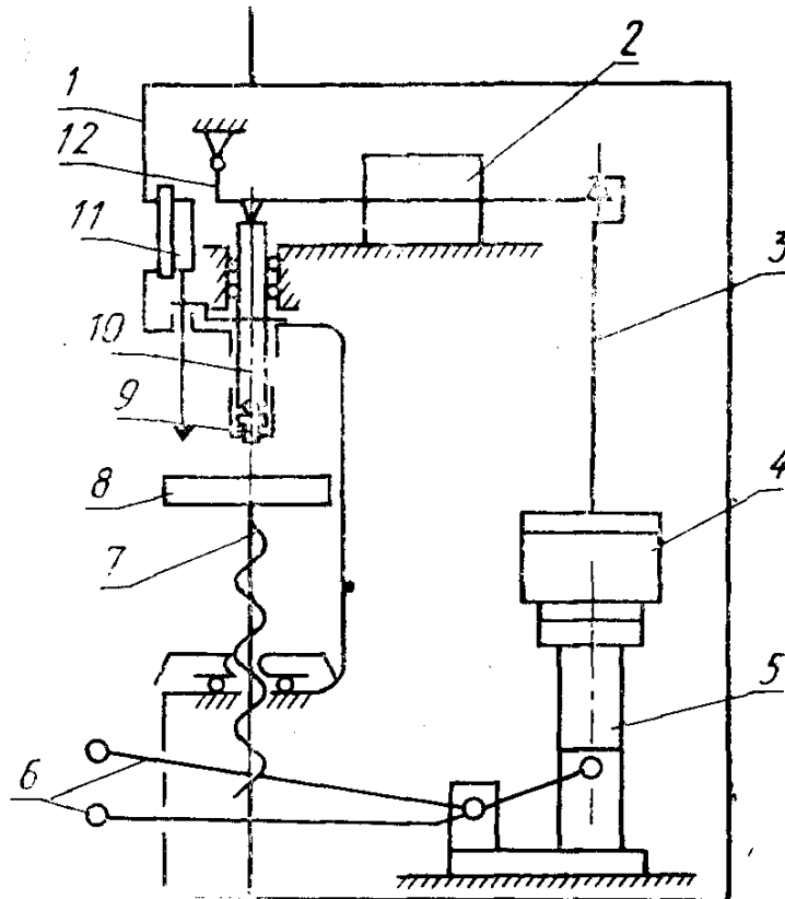
Схема приборов ПСП-67 и ПСП-72
