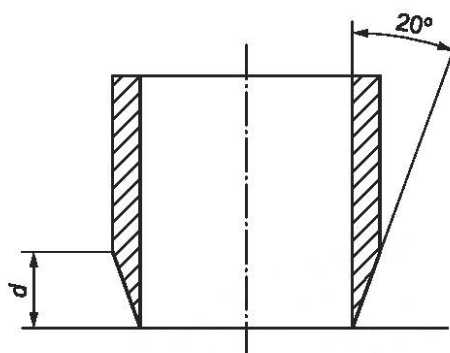
Рисунок 6 — Конструкция резачка
