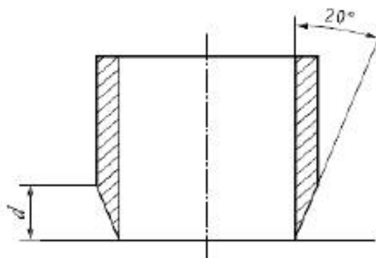
Рисунок 1 – Конструкция резака
