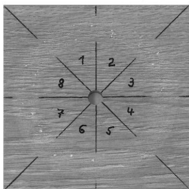
а) Испытание в недостаточном объеме: износ площадью не менее 1,00 \text{ мм}^2 замечен только в октантах 6 и 7
