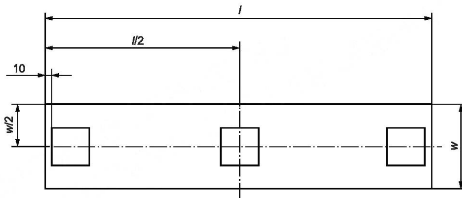
Рисунок 5 — Отбор проб от одного элемента напольного покрытия
