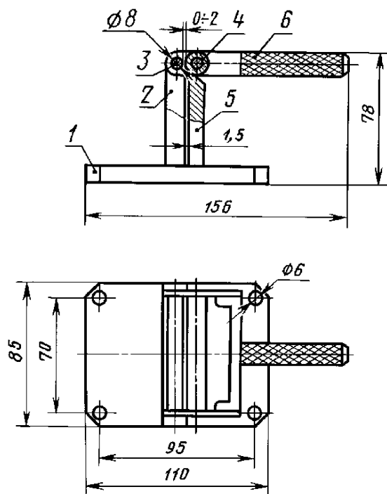
1 — плита; 2 — стойка; 3 — палец; 4 — обойма; 5 — упор; 6 — рукоятка
