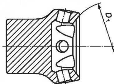
Рисунок 2 — Схематичное изображение адаптера «под пирамиду»
