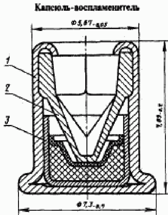
1 — оболочка; 2 — наковальня; 3 — малый капсюль-воспламенитель
